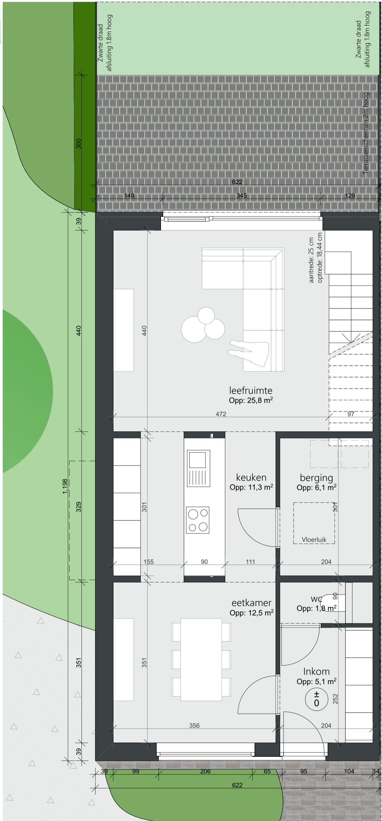
Grond plan: niv +0
