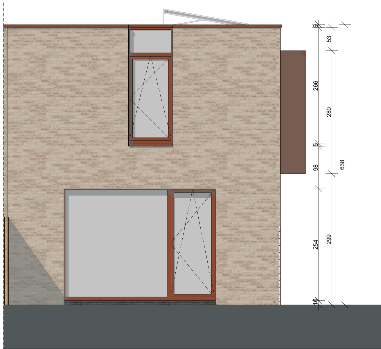
Achtergevel
