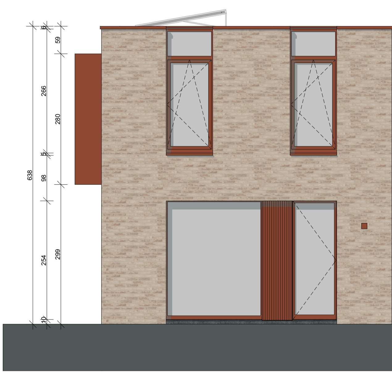
Voorgevel
