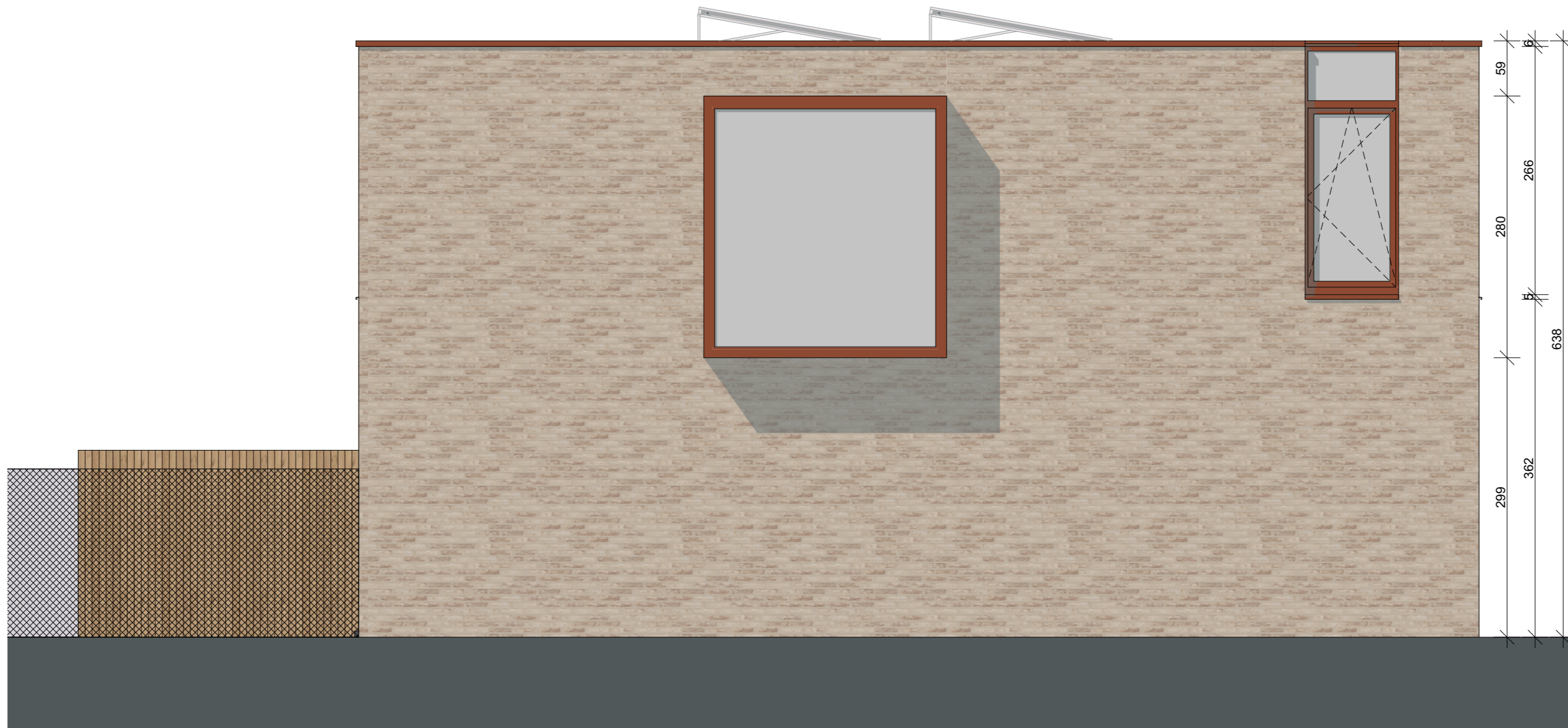
Linker zijgevel
