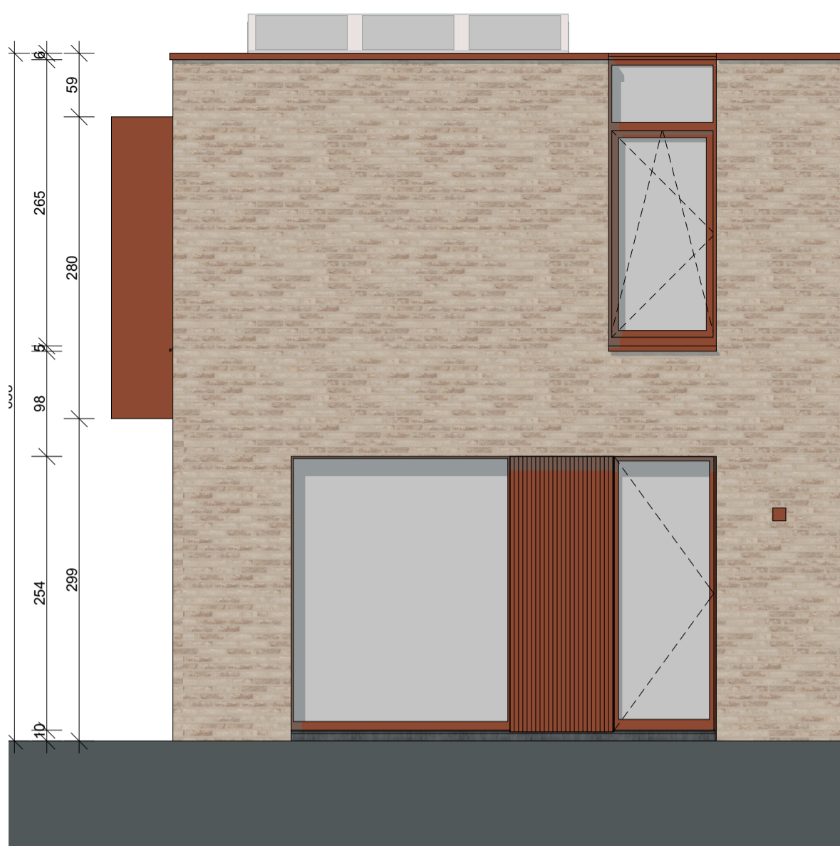
Voorgevel
