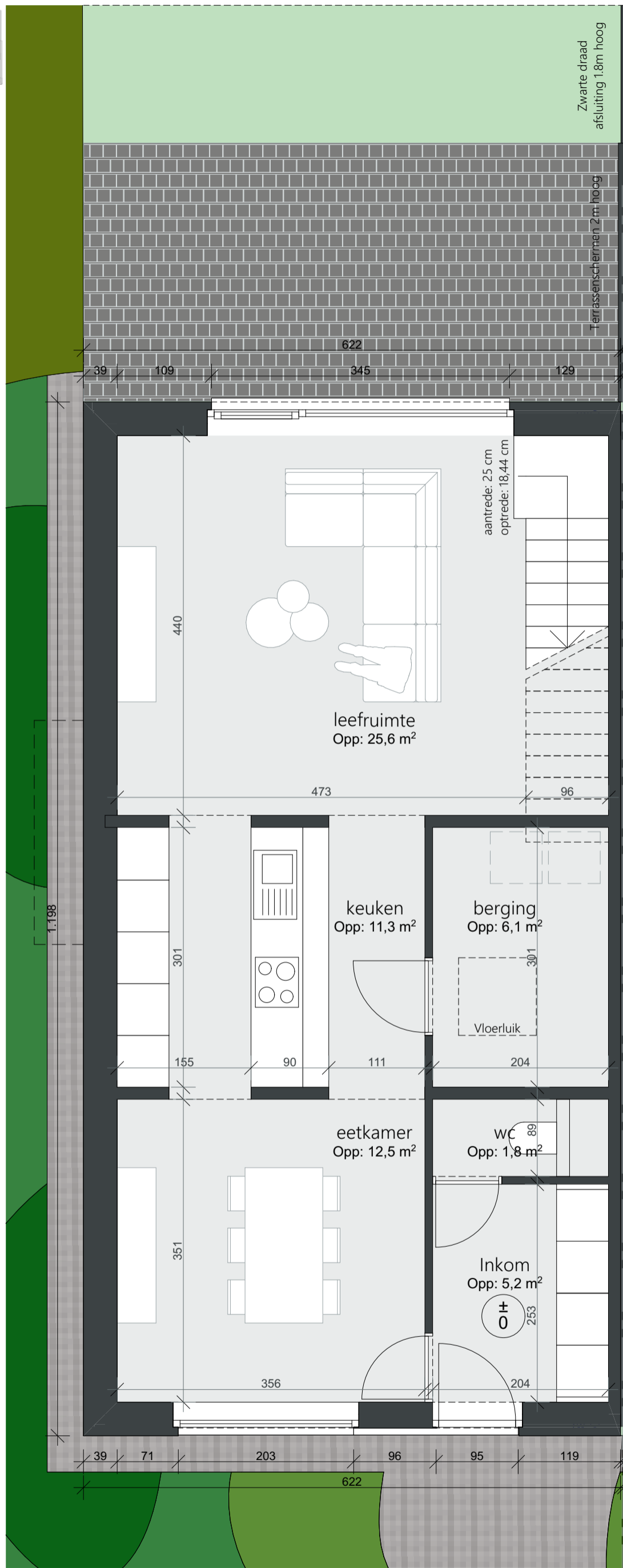
Grond plan: niv +0
